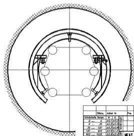
Kreissegmente, Fahrwerk
